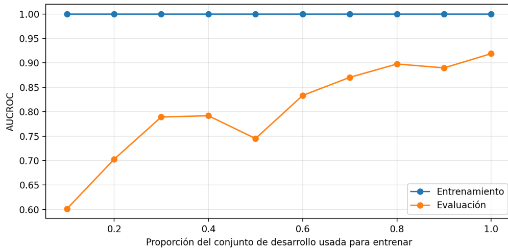
Figura 1: Curva de aprendizaje del SVM polinómico de grado 2: AUCROC sobre entrenamiento y sobre el conjunto de evaluación en función de la proporción del conjunto de desarrollo usada para entrenar.
